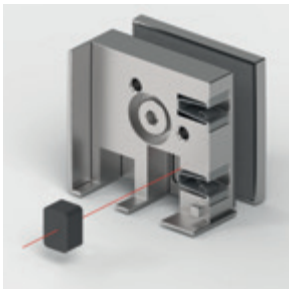
Glashalter am Seitenteil glass bracket on the side panel Art.-Nr.: | art no.: 8822ZN_-GRS/GLS
