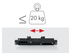
Softstopp doppelseitig (20 kg) softstopp double-sided (20 kg) Art.-Nr.: | art. no.: 8822RAL7016-SSDD-20
