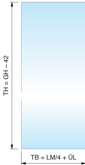
Türflügel door
